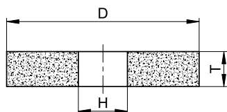
Forma 1 (senza rinforzo)
