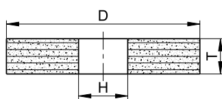
Forma 1F63 (con rinforzo)
